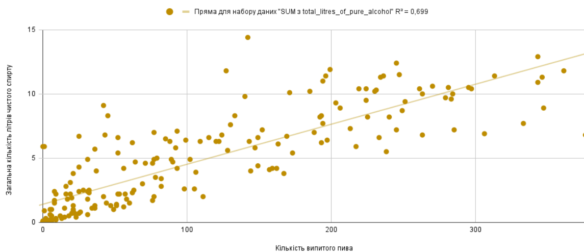
Залежність між загальною кількістю літрів чистого спирту та пива
